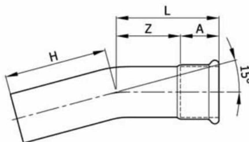
15° M.F. Elbow
