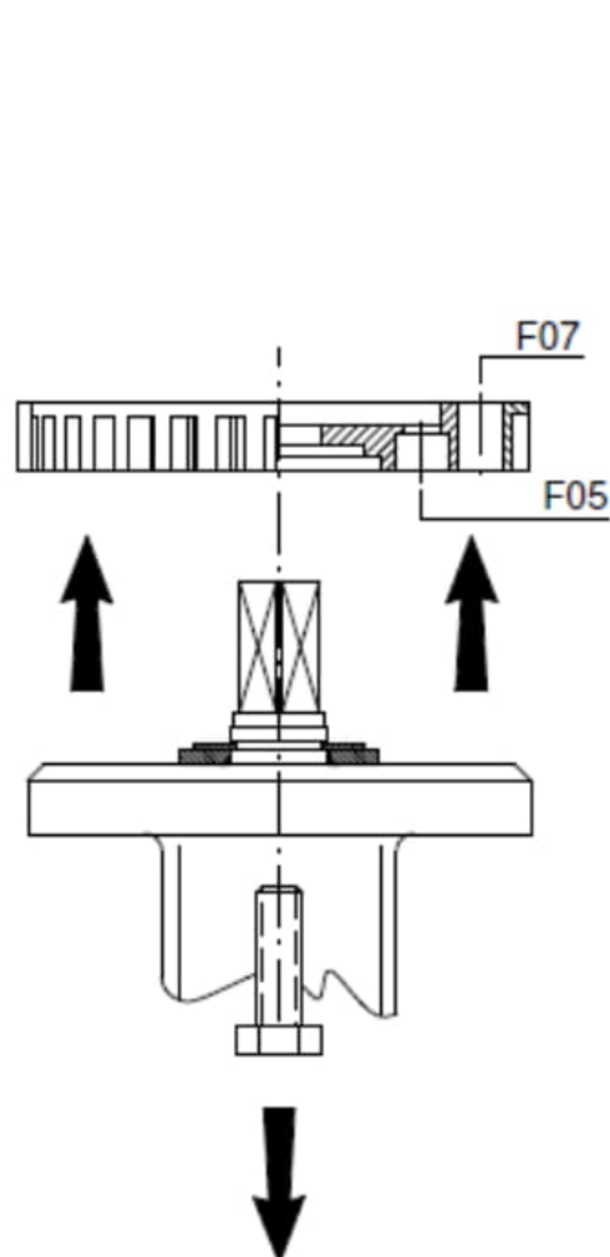
Dévisser et retirer la platine
