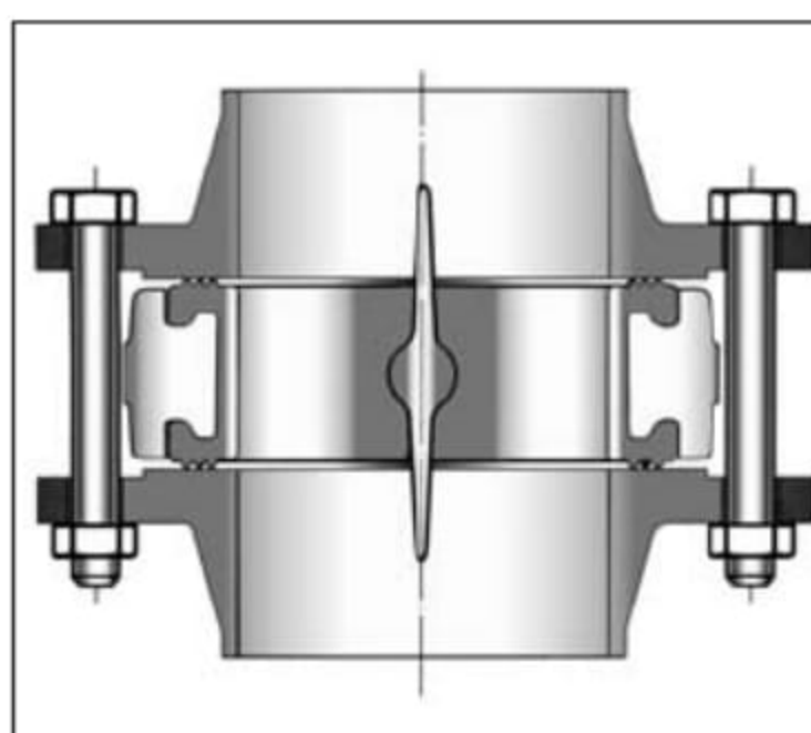
Serrage des boulons robinet ouvert
