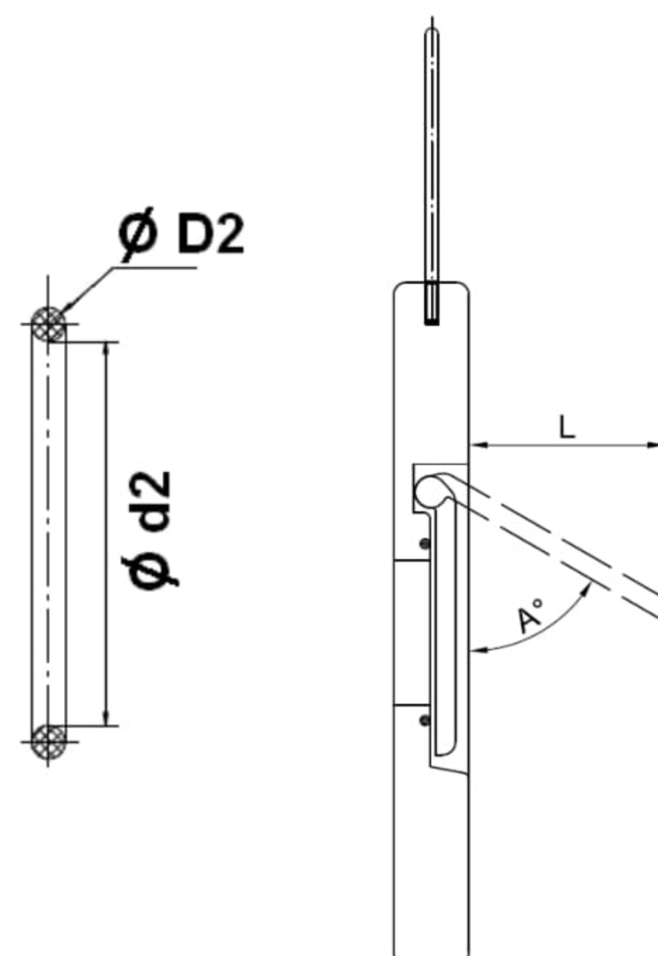
CLAPET OUVERT
