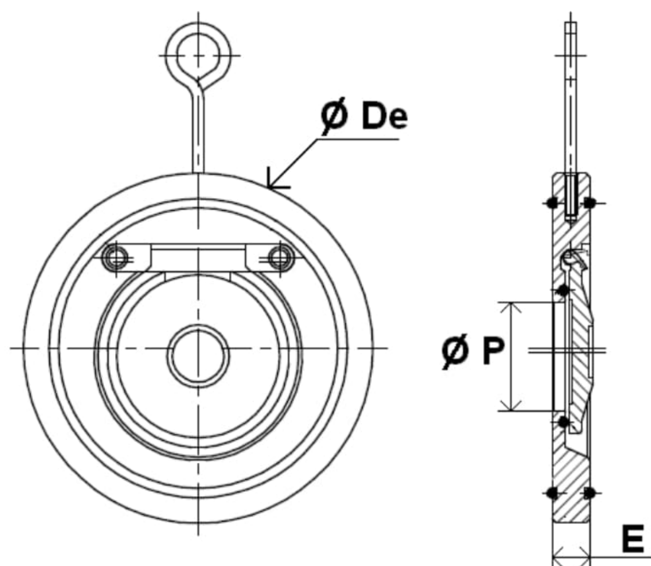
CLAPET FERME
