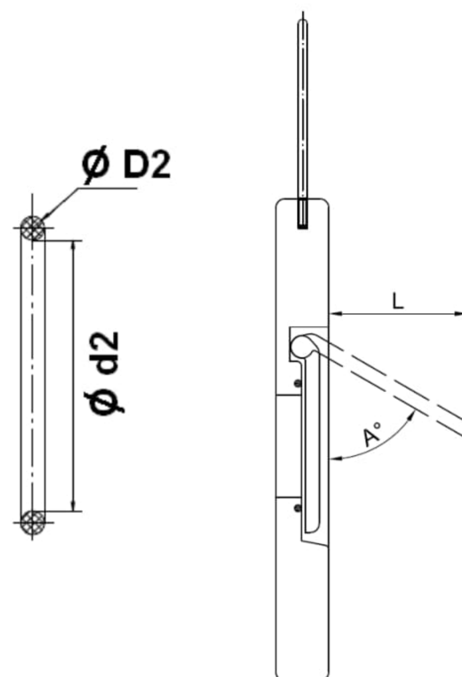
CLAPET OUVERT
