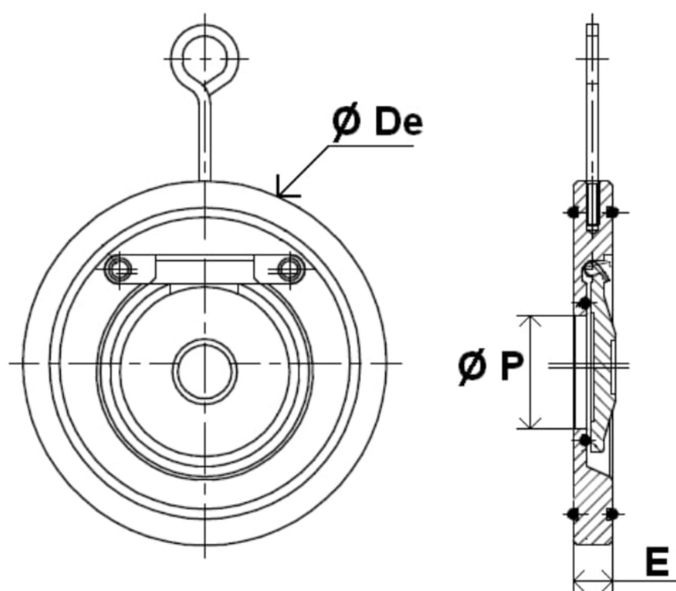
CLAPET FERME
